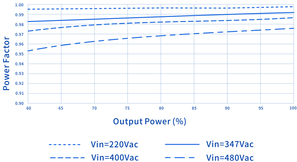
功率因数Vs.输出功率
